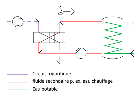
Fig. 2: Illustration simplifiée de l'intégration des accumulateurs à tube en spirale (source ASF)
