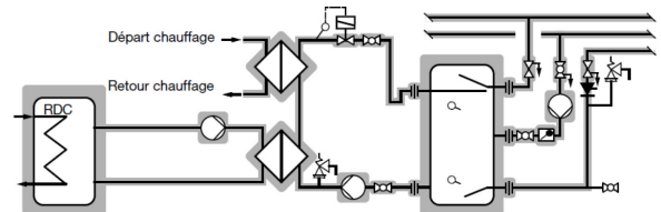
Fig. 37 de la SVGW W3/E3 : Récupération de chaleur à partir de froid commercial dans un accumulateur d'eau industrielle. Production d'eau chaude au moyen d'un échangeur de chaleur externe pour le préchauffage de l'eau potable avec un échangeur de chaleur externe supplémentaire pour agents énergétiques séparés (bois, pompe à chaleur, gaz, mazout, électricité), accumulateur d'eau chaude avec charge stratifiée et soupape d'étranglement avec pompe de charge à vitesse régulée.
